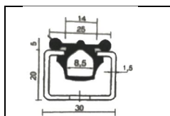
Schalldämmungs-einlegegummi RU 25
